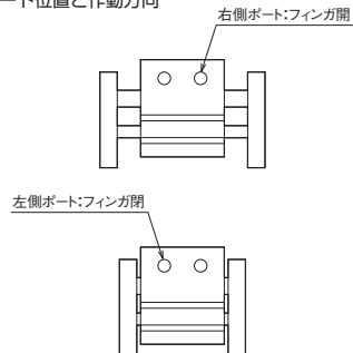
●配管ポート位置と作動方向
