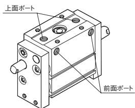
●配管ポート位置と作動方向
