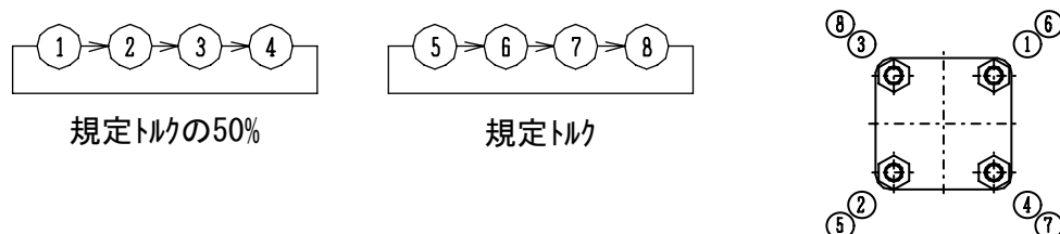
タイロッド締め付け規定トルク表（モリブデンペーストによる潤滑時）：T C形以外
