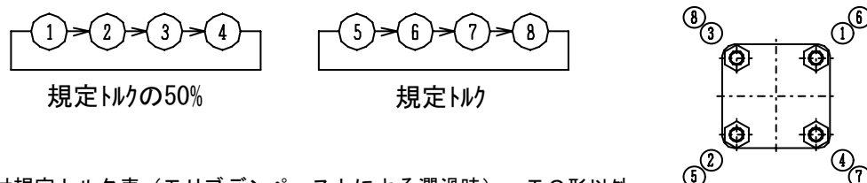
タイロッド締め付け規定トルク表（モリブデンペーストによる潤滑時）：T C形以外
