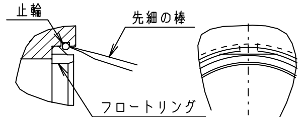
ロッドカバー側フロートリング
