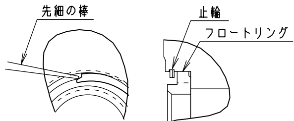
ヘッドカバー側フロートリング
