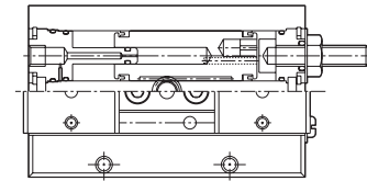
上図は閉側調整付の図です。
