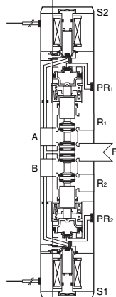
SR552-CN2 (ソレノイドS1、S2とも非通電)
