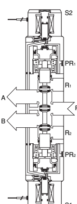
SR562-PN3 (ソレノイドS1、S2とも非通電)
