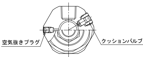
〔空気抜きプラグの位置〕
