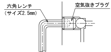
〔空気抜きプラグの詳細図〕
