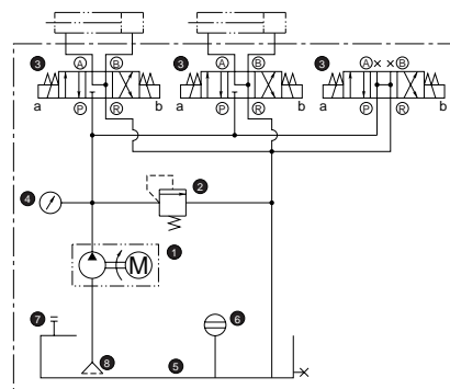
油圧回路 (例)
