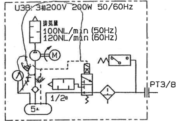
真空回路図
